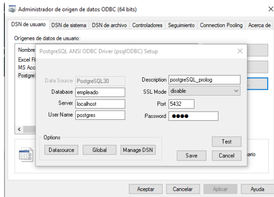
Figura 2: Muestra la configuración del ODBC.
